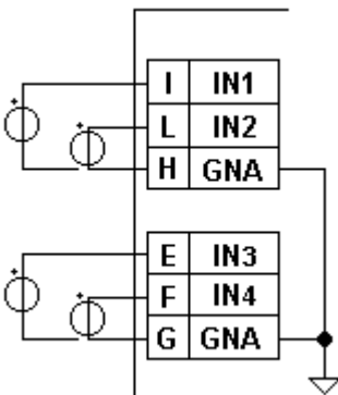
mV wiring
