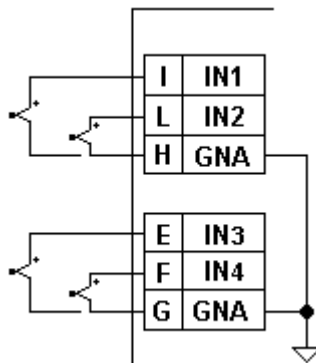
Tc wiring
